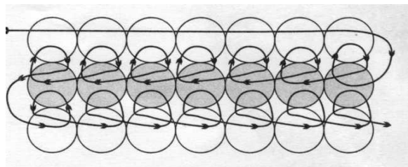
Рис. 1. Плетение прямого полотна
